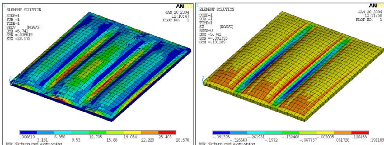
Figur 15: Von Mises spenningene i huden er maksimalt 28 MPa. Trykkspenningene \sigma_z i skummet er oppe i 0.39 MPa dvs 33 % av brudd. Begge disse parameterne er tilfredsstillende.
