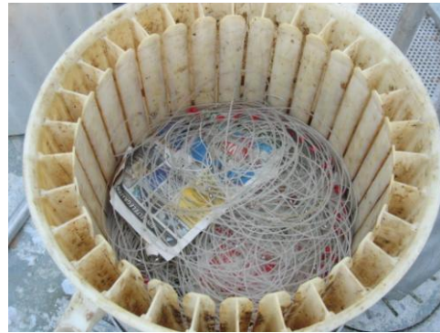
Turboline egne- og krokfesteprensipp (til venstre) og Turboline linestamp med krokkammer till høyre.
