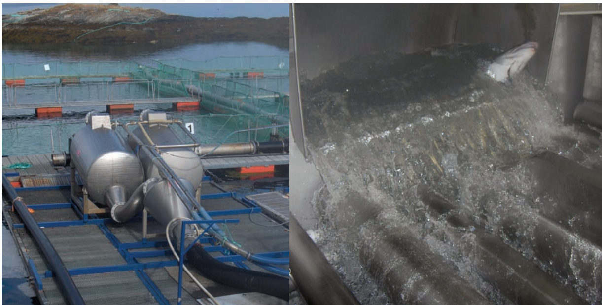
Figur 27. Slakteri C. Bildet til venstre viser ventemerder og dobbel vakuumpumpe plassert på flytebrygge, som gir lav løftehøyde i sugefasen. Bildet til høyre viser laks på vei inn i avsilingen der fisken størrelsessorteres. Mindre fisk faller mellom rørene og ledes til annen rigg enn den større fisken.
