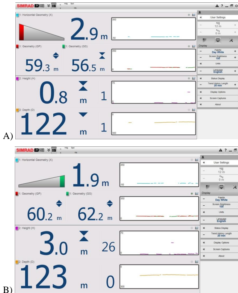
Figur 2.4.10. Skjerm bilde av A) litt skeiv snurrevad med babord vingelitt foran styrbord vingel, fiskelinen 0.8 meter over bunnen (samme høyde som skjørt; snurrevad følger bunnen). B) Styrbord vingelitt foran babord vingel, Snurrevad har løftet seg fra bunnen, fisk som står foran redskapen ned ved bunnen vil unnslippe under skjørtet. Begge skjerm bildene fra samme hal (se tidslinjer på A og B).
