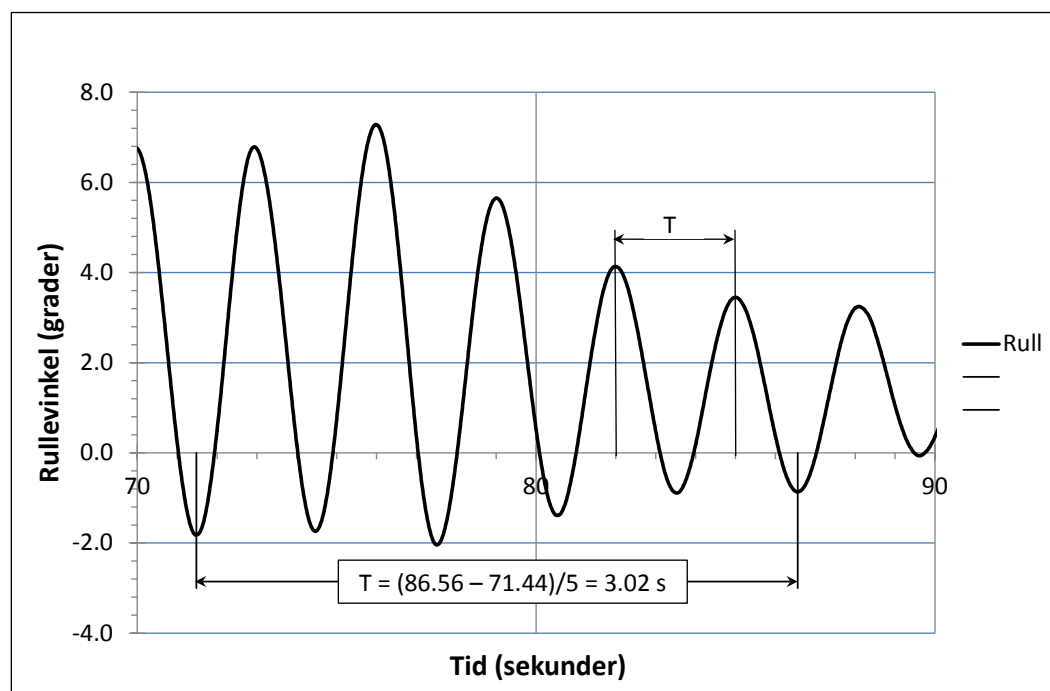
Figur 4 Egenrullesvingninger, Test 01 (før avgang)
