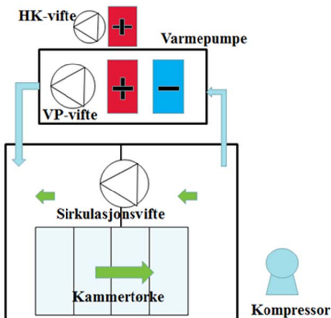
Figur 4: Kammertørke med varmepumpeaggregat i by-pass. Deler av sirkulert luftmengde i kammer blir avfuktet vha. varmepumpe. (Har erstattet de fleste Portugaltdørkene som var installert tidligere)
