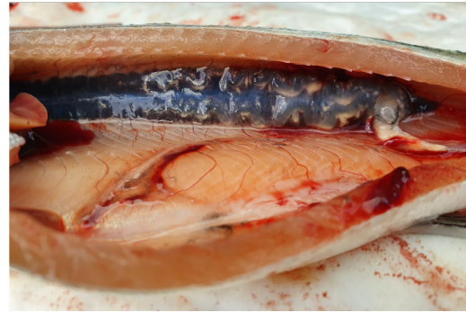
(d) Score 4.
